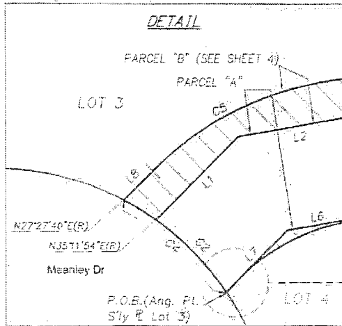
SCALE: 1" = 20'
